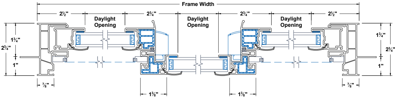
Jambs
