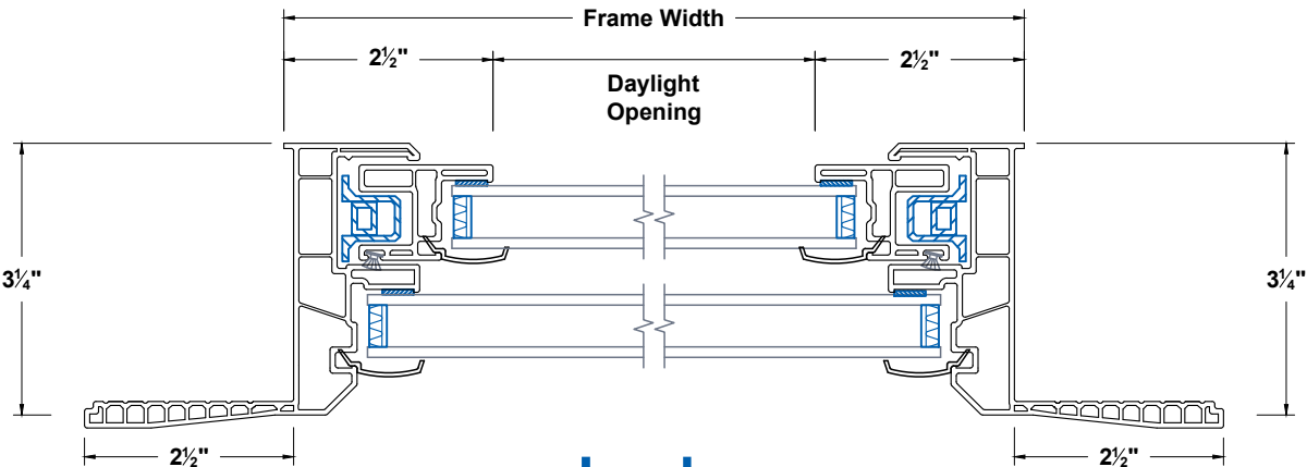
Jambs
