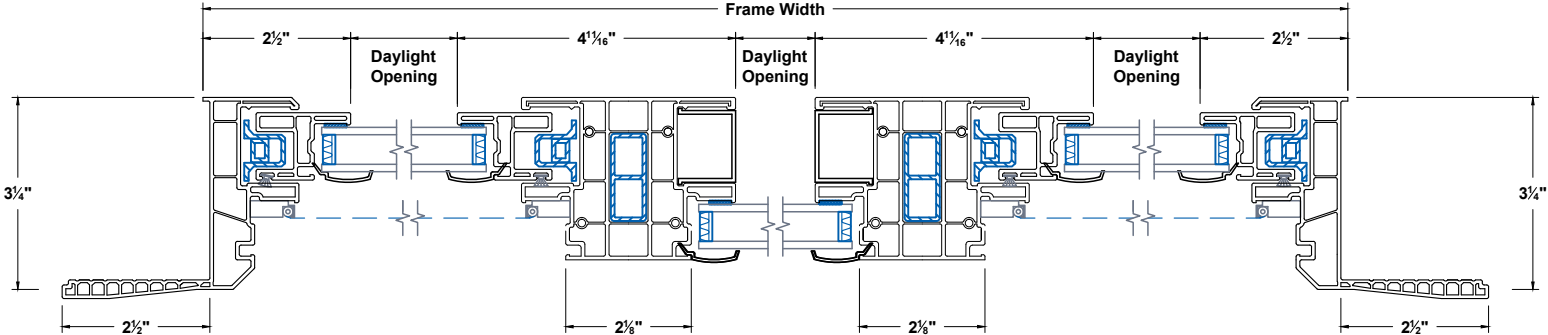
Jambs
