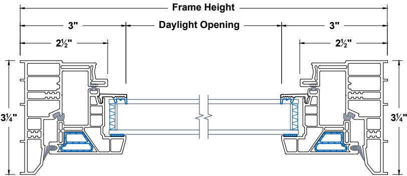
Jambs
