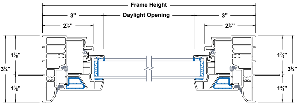
Jambs
