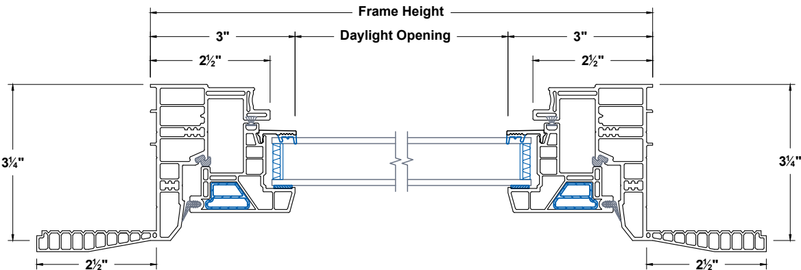
Jambs
