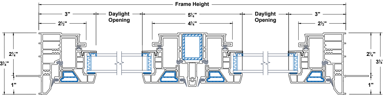
Jambs
