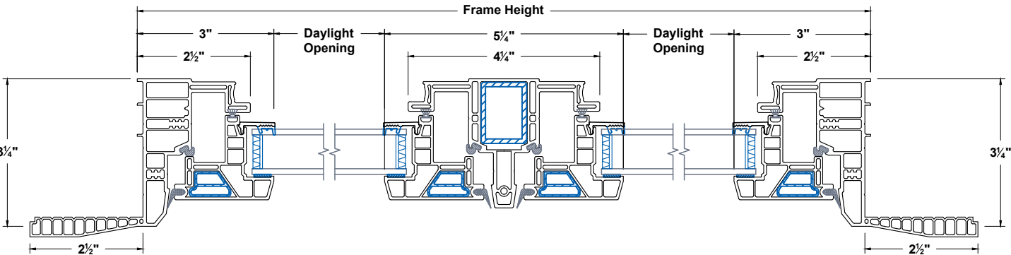
Jambs
