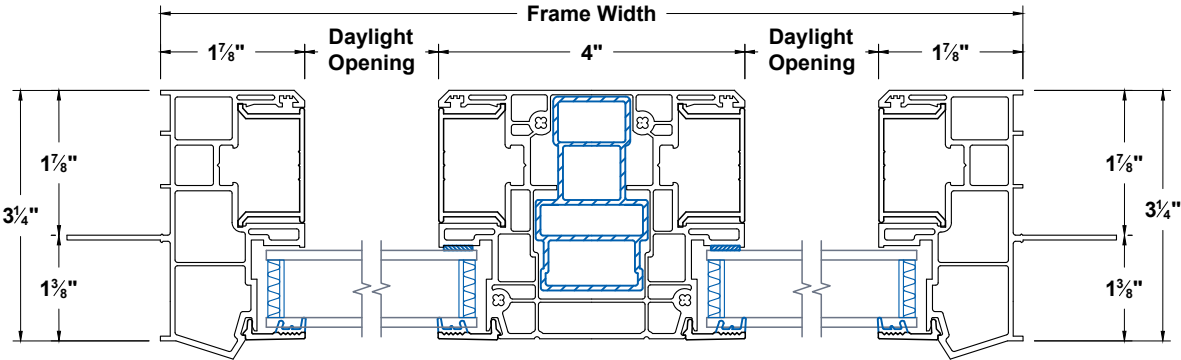
Jambs
