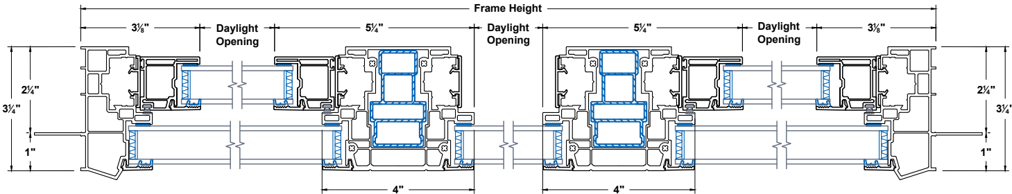
Jambs
