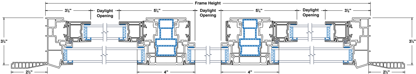
Jambs
