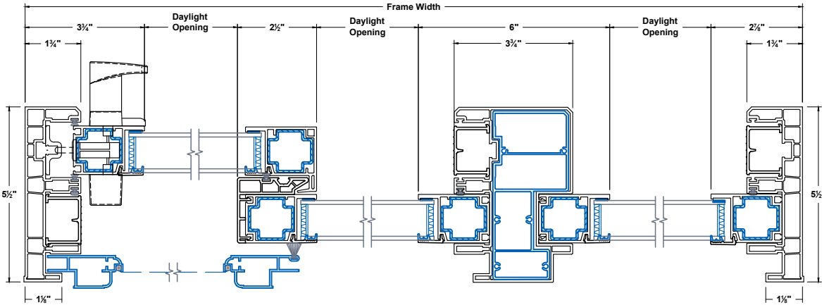
Jambs
