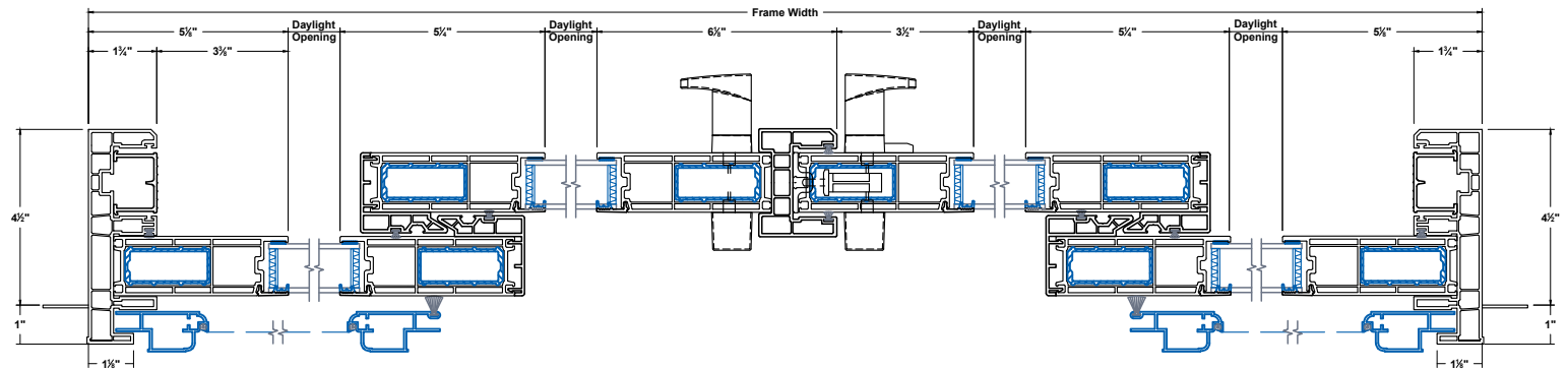
Jambs
