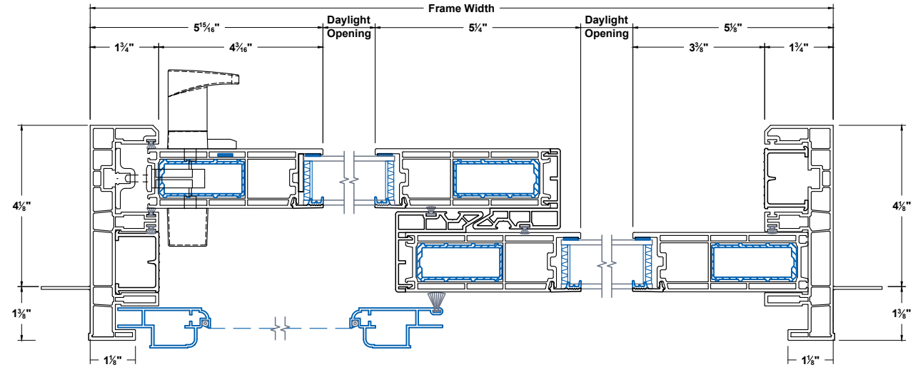
Jambs
