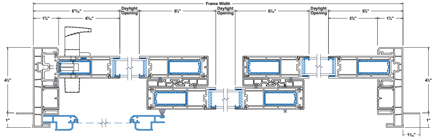
Jambs
