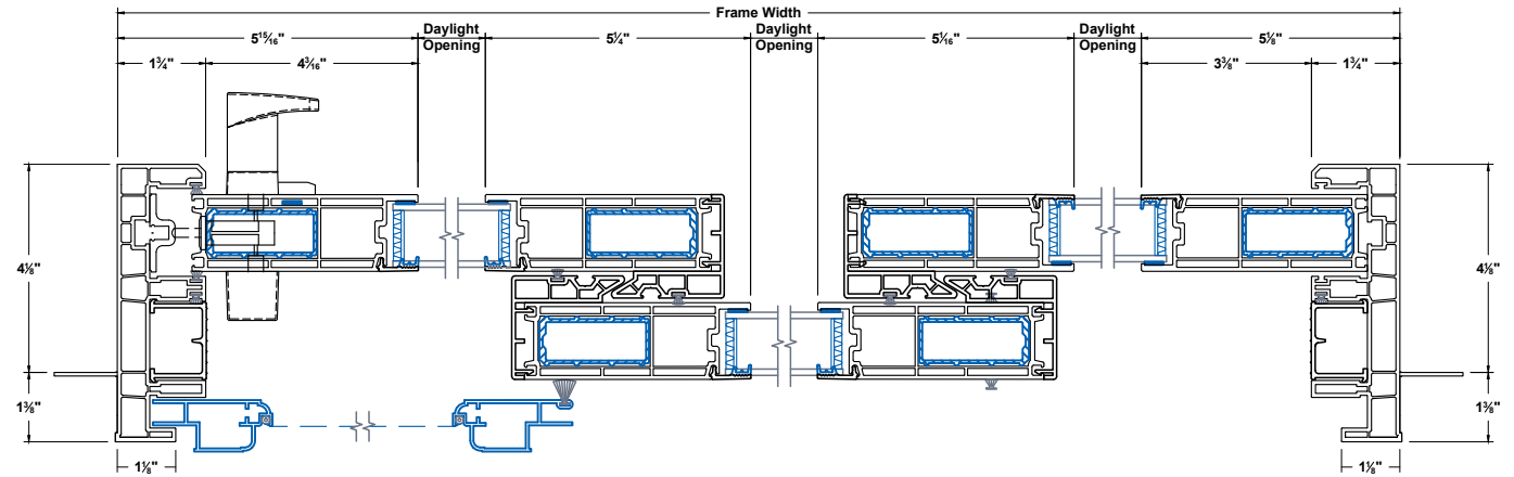
Jambs
