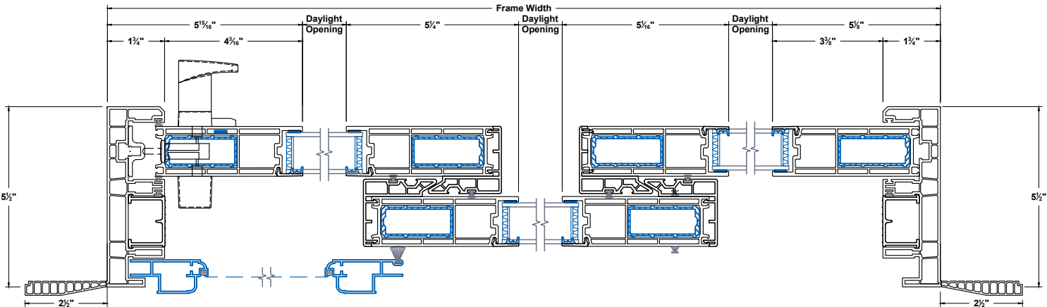
Jamb
