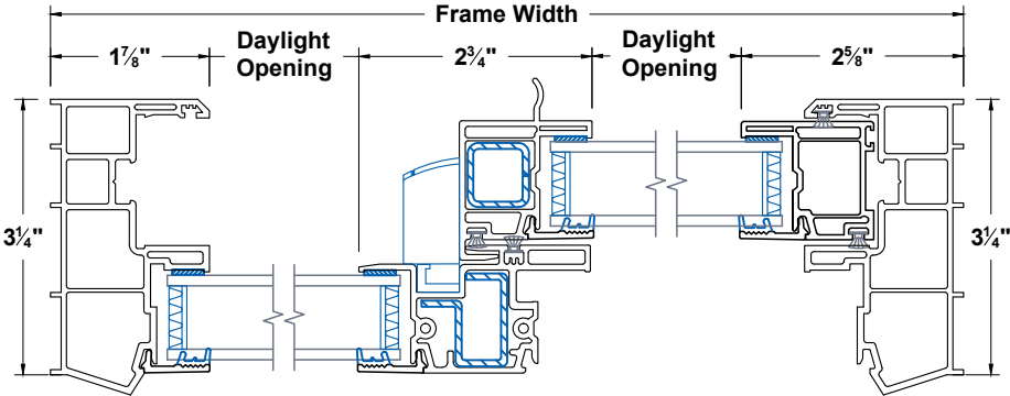
Jambs
