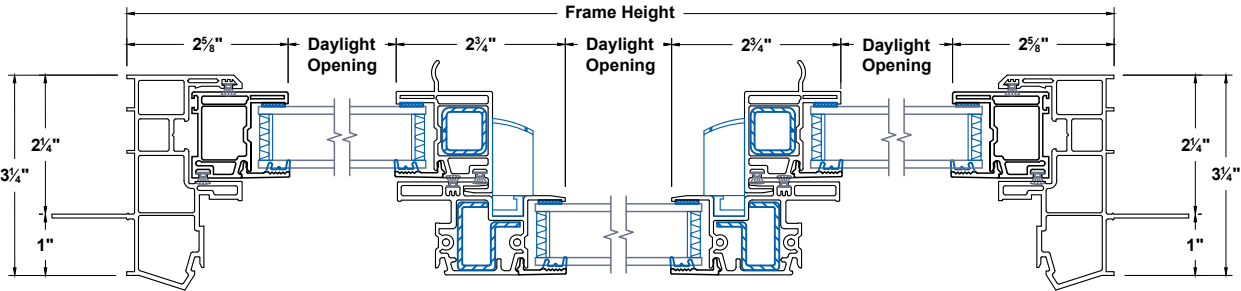
Jambs
