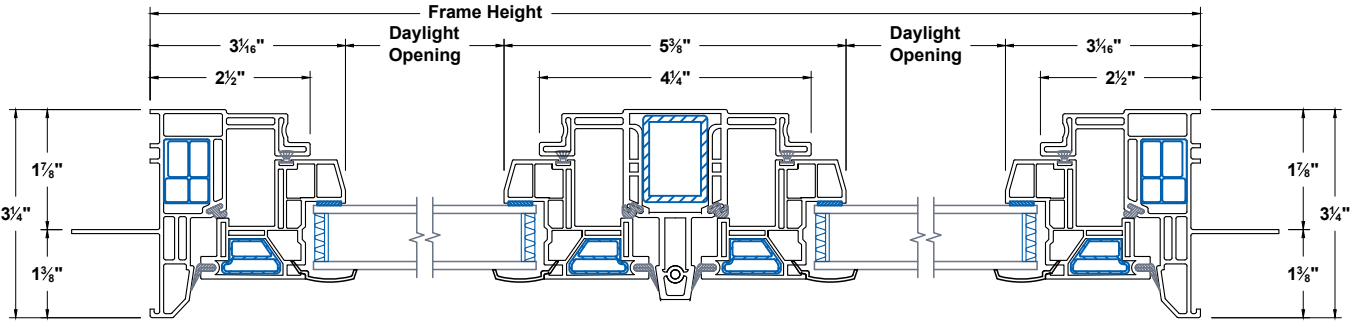
Jambs
