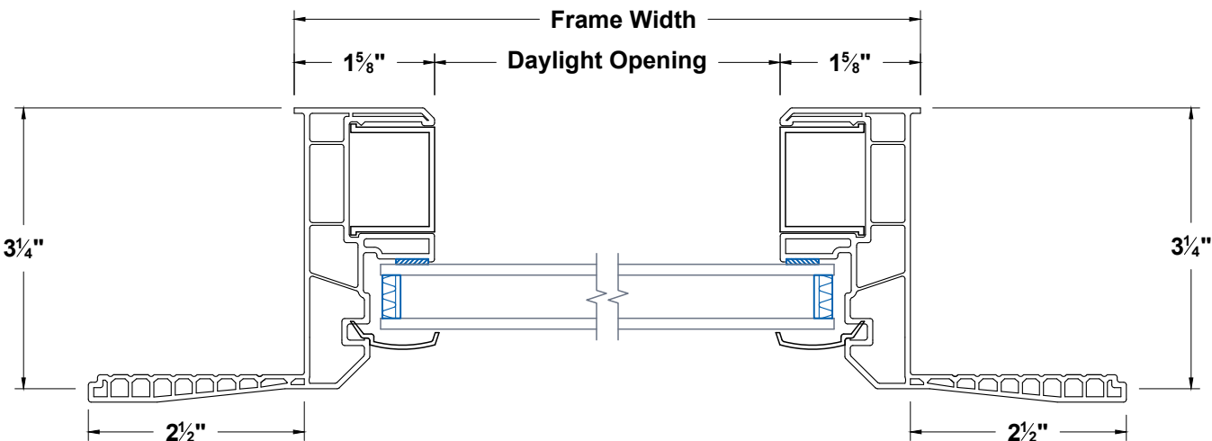
Jambs
