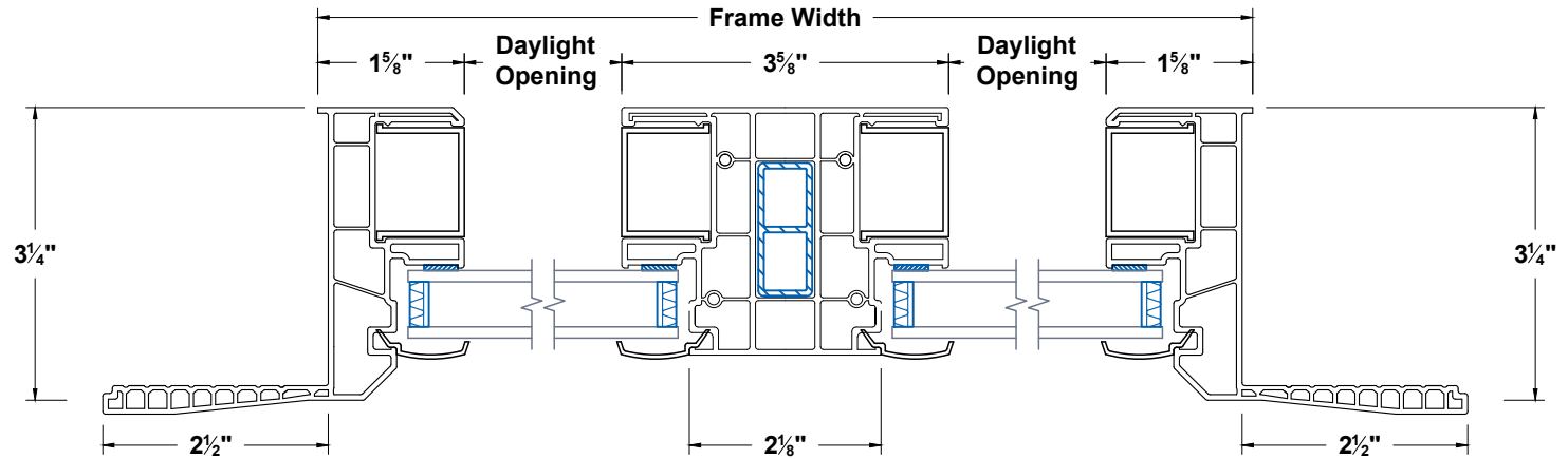
Jambs
