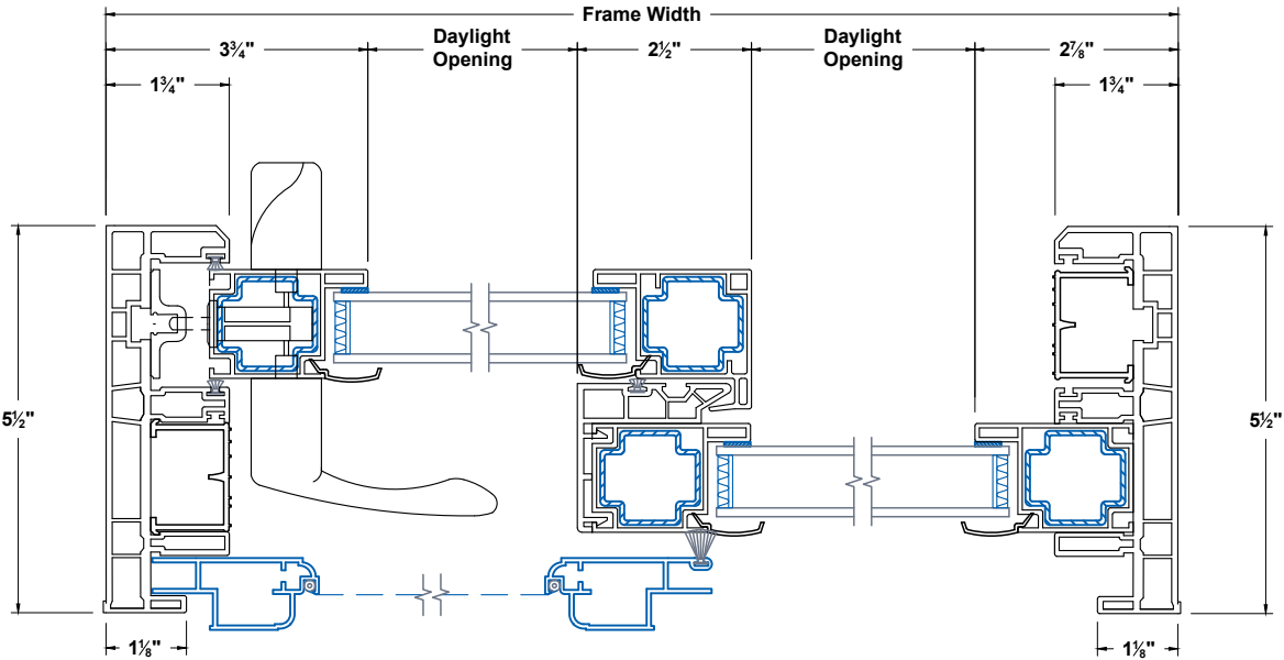
Jambs
